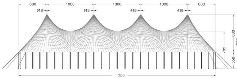
Zijaanzicht
