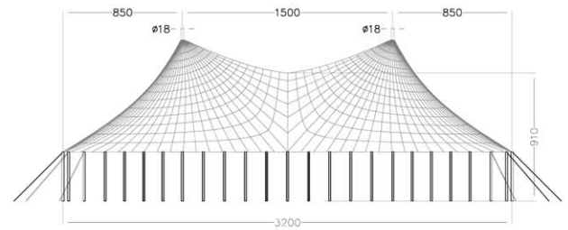
Vooraanzicht
